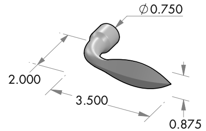
L-16 Mini Quigley lever.
