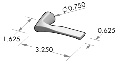
L-54RH Mini Galena lever. Right hand.
