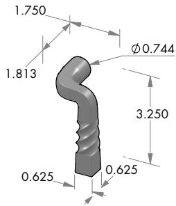
L-23OH-RH Mini Twist lever. Right hand.
