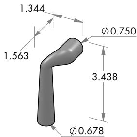
L-19OHLH Mini Muldoon lever. Left hand.
