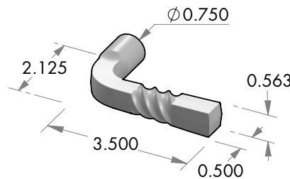
L-23RH Mini Twist lever. Right hand.
