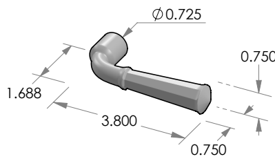
L-28 Mini Stanley lever.
