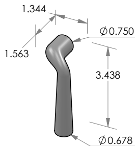
L-19OHRH Mini Muldoon lever. Right hand.
