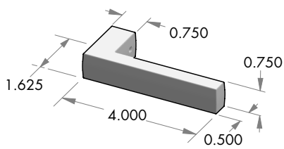
L-67SQ Mini Elle lever.
