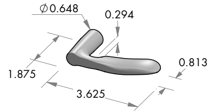
L-26RH Mini Silver Creek lever. Right hand.
