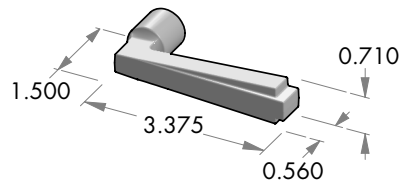
L-42 Mini Deco lever.
