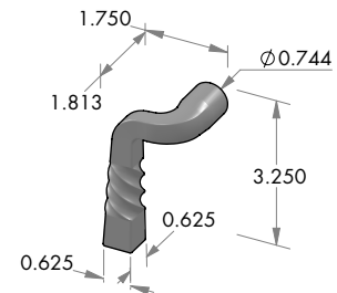
L-23OHLH Mini Twist lever. Left hand.
