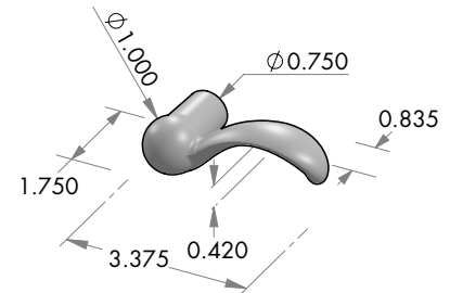
L-20RH Mini Croy lever. Right hand.
