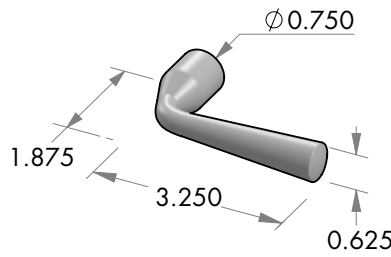
L-13/19 Mini Alturas/Muldoon lever.
