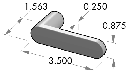
L-11 Mini Flat lever.
