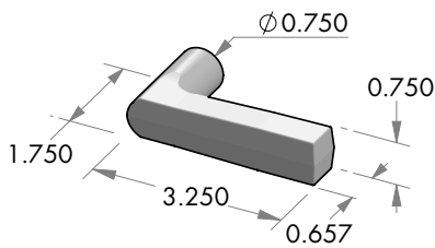
L-22 Mini Metro lever.
