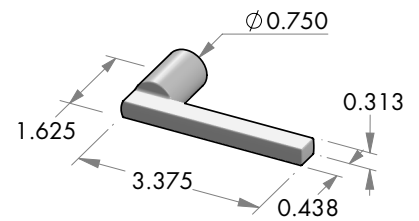
L-29 Mini Della lever.
